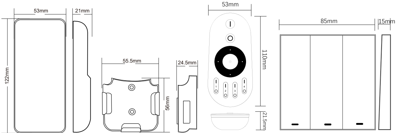
分组简易遥控器
