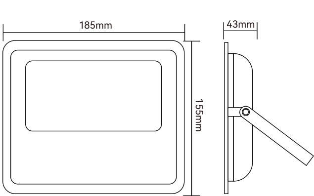
ML30X-30W尺寸
