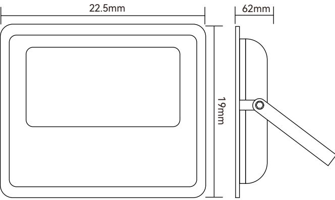
ML30X-50W尺寸
